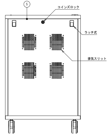
背面図
