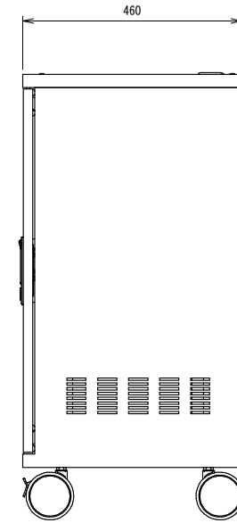
側面図
