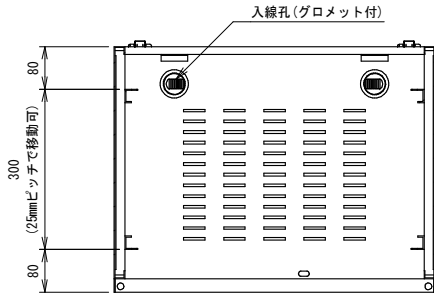
断面図AA
