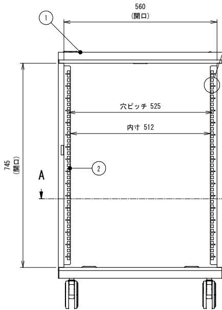
開口図
