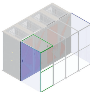
コンテインメントトンネル設置イメージ(3D)
