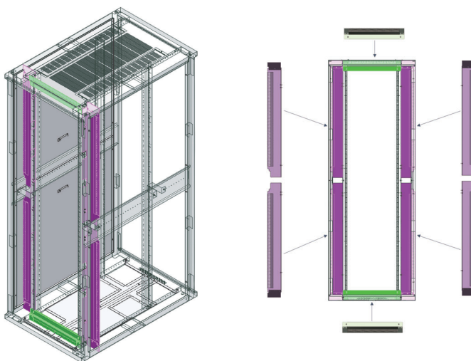
グリーンとピンク部分設置イメージ(3D)
