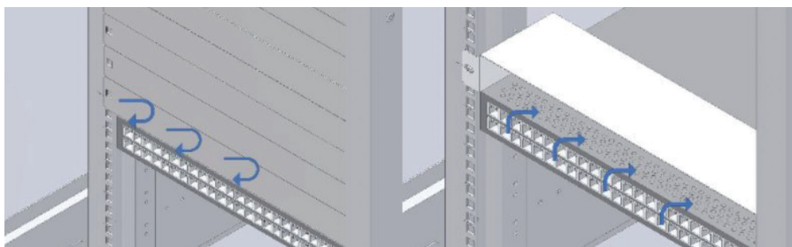
ブランクパネル(左) とブランクトレイ(右) の取付時エアフローイメージ
