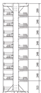
断面図 C-C
