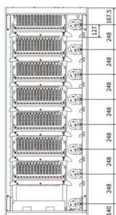
正面図
