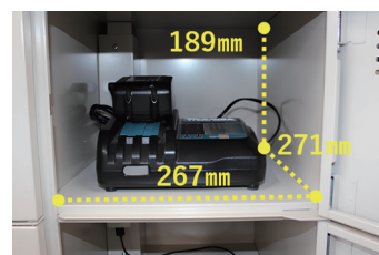
庫内寸法
