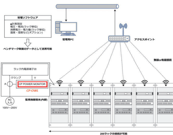
監視システム イメージ図
