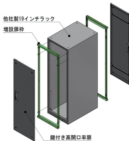
設置イメージ(3D)
