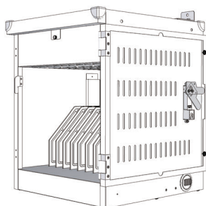
【PCV101-D1-200】 10台収納タイプ
