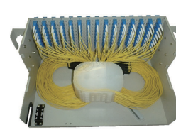
融着BOX(内部)
