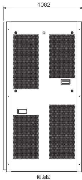
側面図
