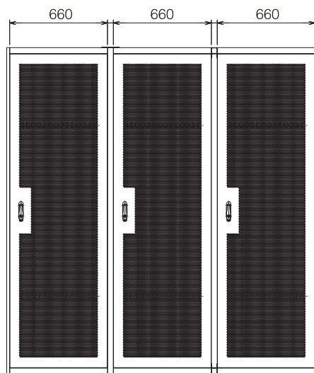
正面図
