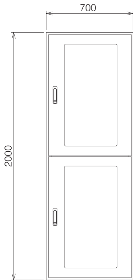
正面図
