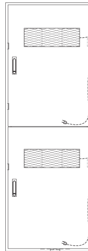
背面図
